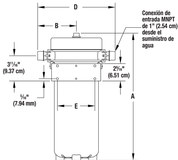
Vista posterior
